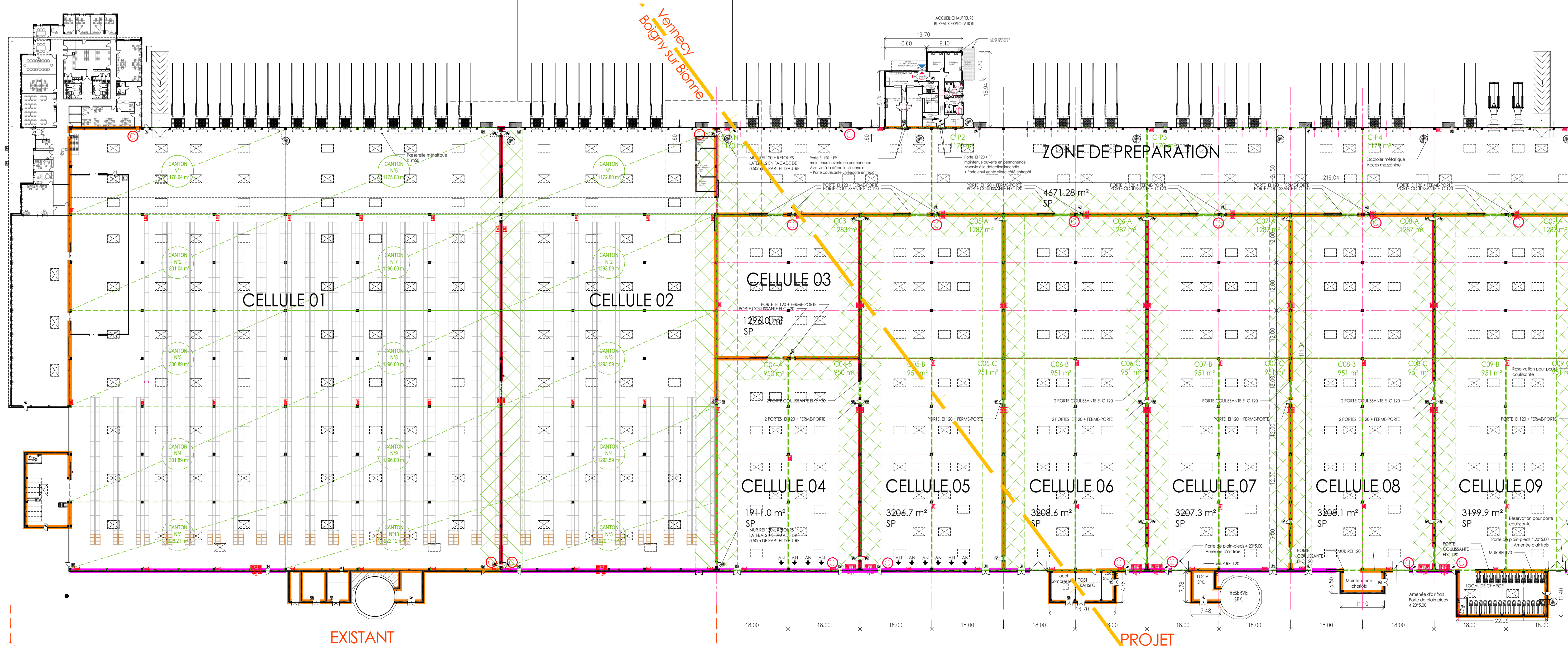
EXTRAITS NIVEAU MEZZANINE Ech : 1/500
