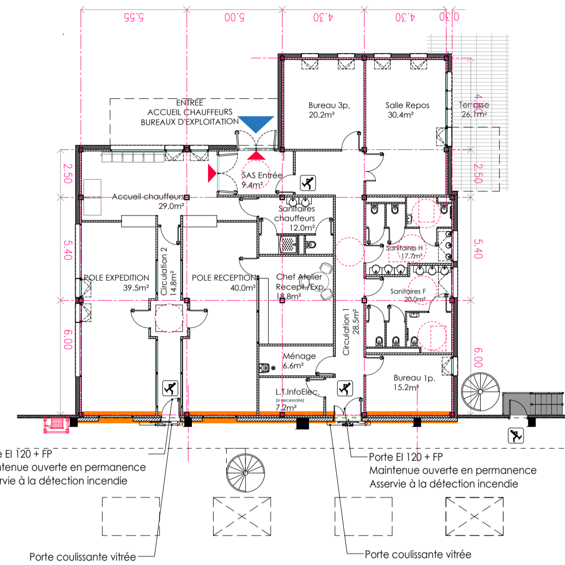
ACCUEIL CHAUFFEURS ET BUREAUX DE QUAIS Ech : 1/200
